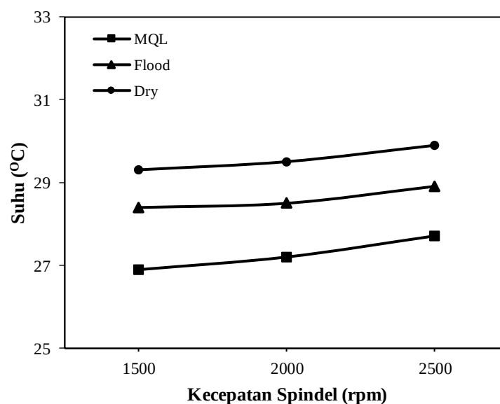
Gambar 6. Hubungan antara parameter pemotongan terhadap suhu
