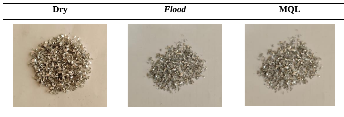
Gambar 7. Morphology tatal di bawah lingkungan milling yang berbeda.
