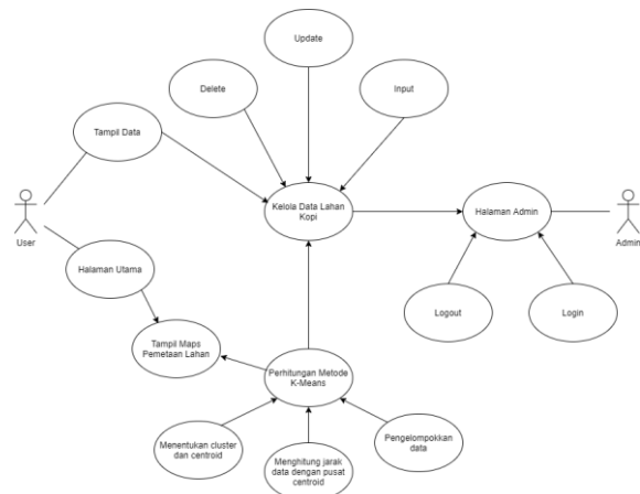
Gambar 1. Use Case Diagram Pemetaan Lahan Kopi
