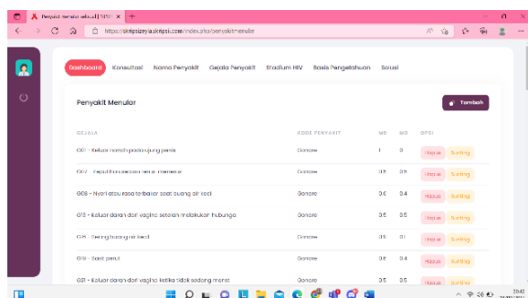
Gambar 11. Halaman Gejala
