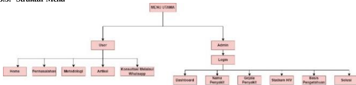
Gambar 2. Struktur Menu
