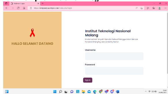
Gambar 9. Halaman Login
