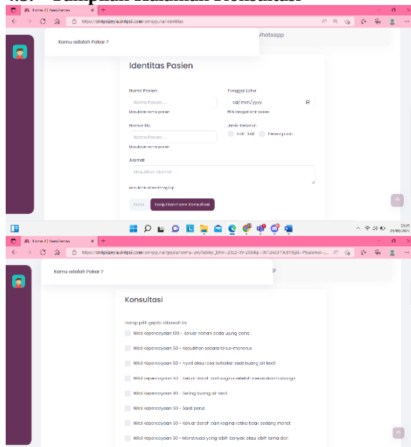
Gambar 8. Halaman Konsultasi
