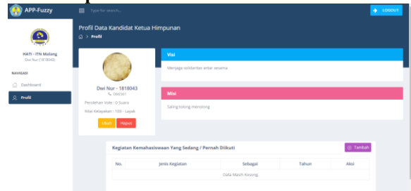
Gambar 15. Halaman Profil
