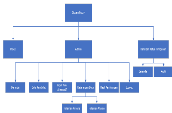
Gambar 8. Struktur Menu.
