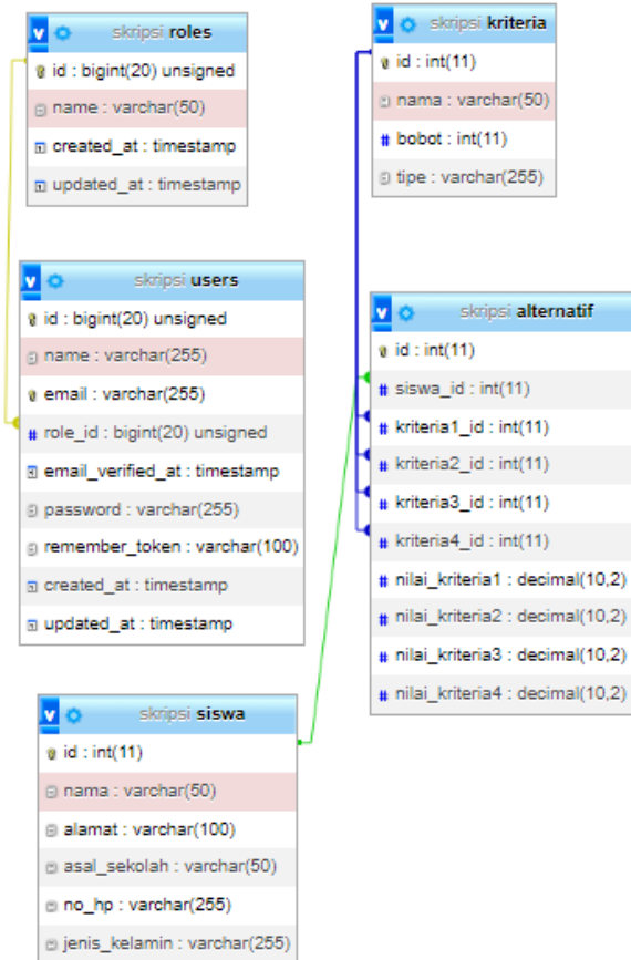
Gambar 3. Relasi Tabel Database
