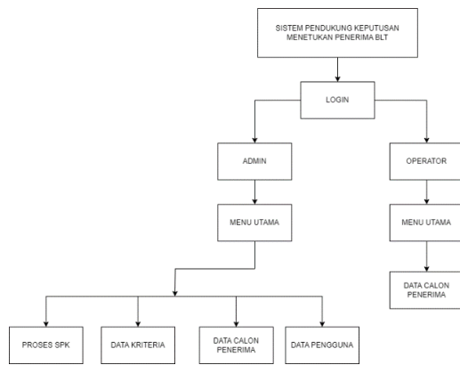
Gambar 2. Struktur Menu
