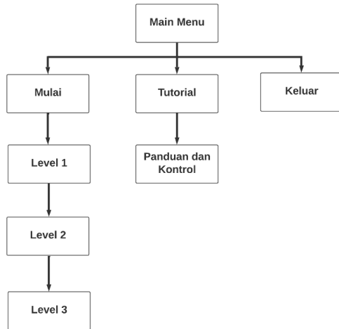
Gambar 3. Struktur Menu
