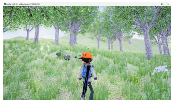
Gambar 7. Map
