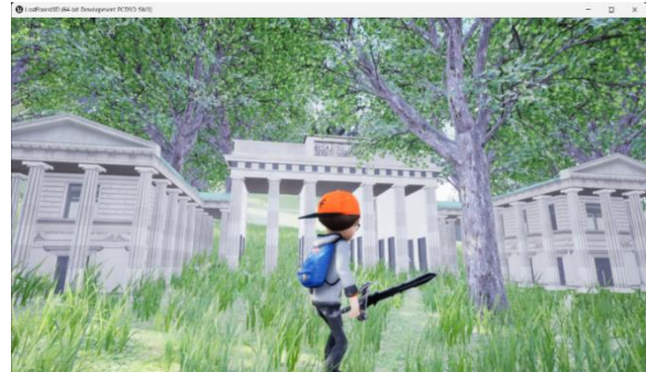
Gambar 13. Bangunan Kuno
