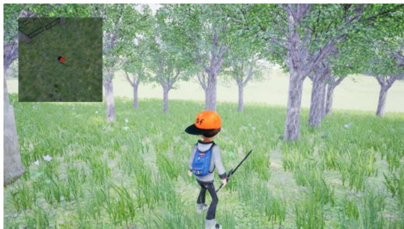
Gambar 11. Mini Map
