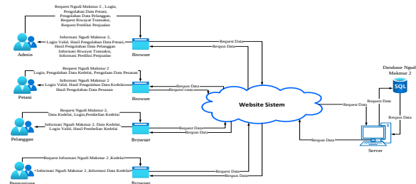
Gambar 2. Desain Sistem
