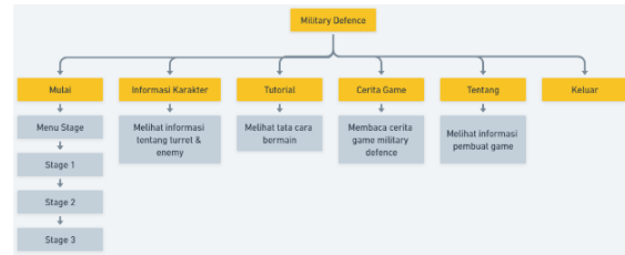
Gambar 3. Struktur Menu
