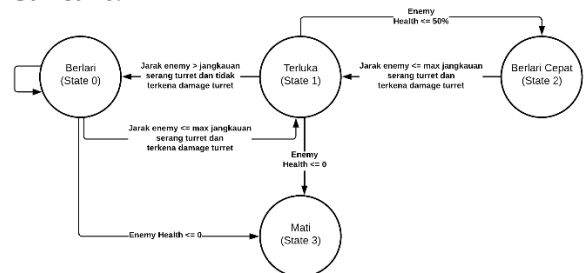
Gambar 6. Alur FSM pada Enemy Moster Sword
