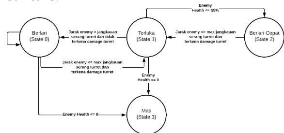
Gambar 5. Alur FSM pada Enemy Moster Green
