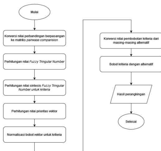
Gambar 5. Tahapan fuzzy
