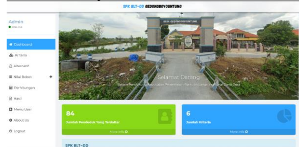
Gambar 9. Halaman dasbor
