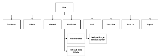
Gambar 7. Struktur menu
