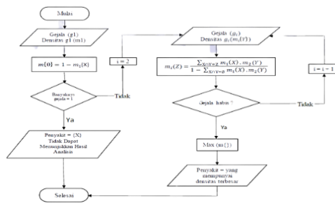
Gambar 1. Penerapan rumus
