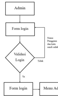
Gambar 1. Struktur Menu
