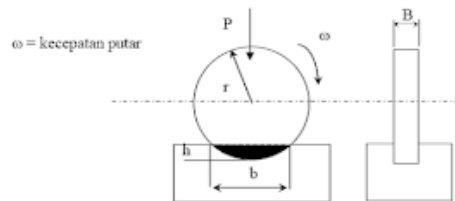
Gambar 4. Pengujian Keausan Dengan Metode Ogoshi
