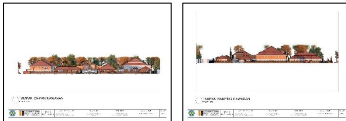
Gambar 19. Tampak Depan (kiri) & Tampak Samping (kanan) Sumber: Analisa, 2023
