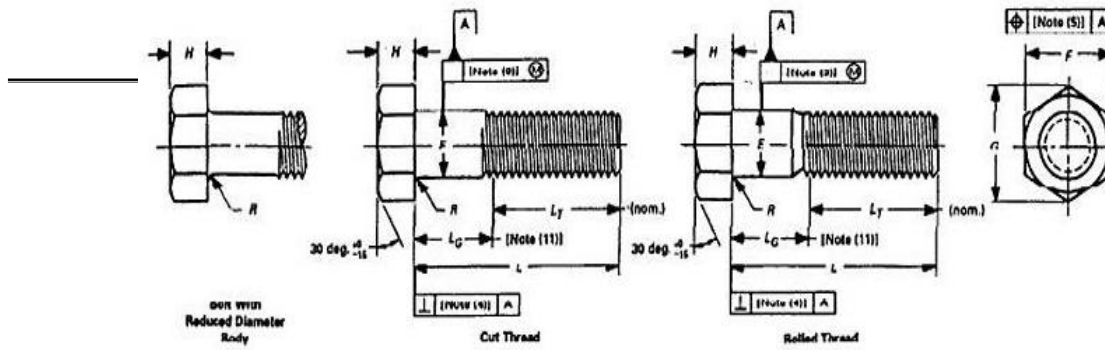
Gambar 2.3 Spesifikasi Baut A325
