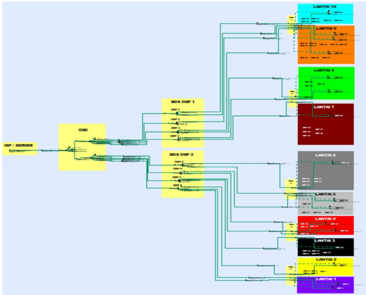
Gambar 2. Rancangan FTTH OptiSystem
