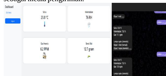
Gambar 9. Notifikasi Telegram
