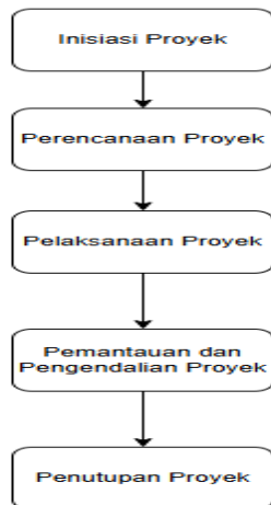
Gambar 1. Tahapan penelitian
