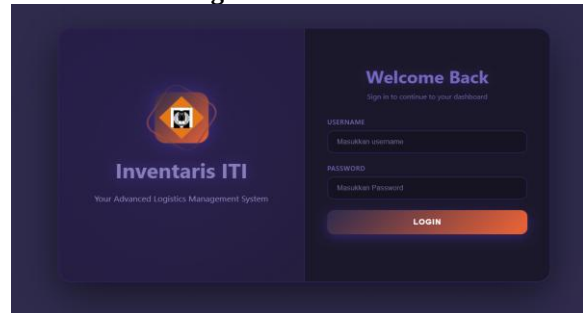
Gambar 8. Halaman login
