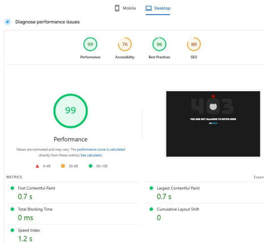
Gambar 11. Pengujian performa
