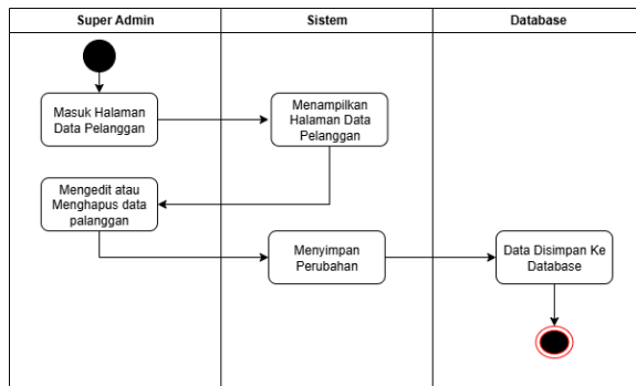
Gambar 5. Diagram Activity Super admin Update Dan Hapus Data Pelanggan
