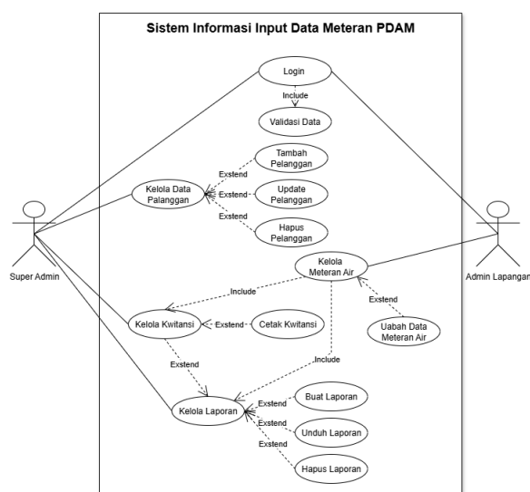
Gambar 2. Use case sistem informasi PDAM
