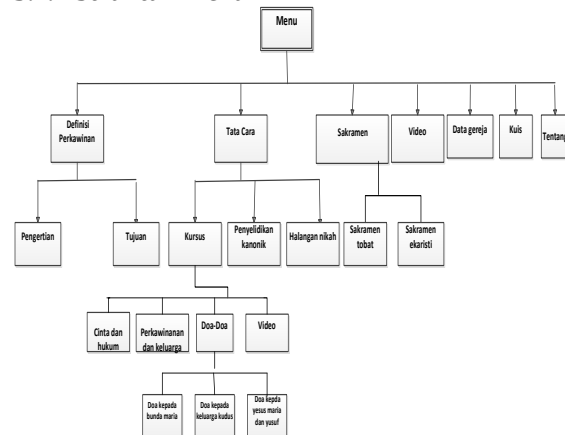
Gambar 3.2.1. Struktur Menu
