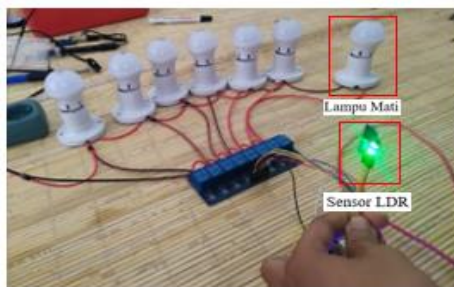
Gambar 7. Pengujian sensor ldr pada cahaya terang
