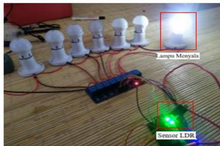
Gambar 8. Pengujian sensor ldr pada cahaya gelap
