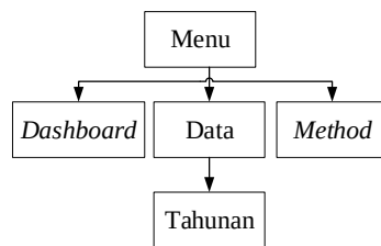
Gambar 2. Struktur menu
