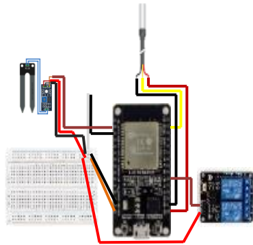
Gambar 10. Rangkaian Skematik Smart Farming Sumber: (Dokumen Pribadi, 2024)
