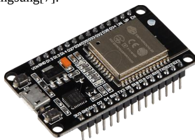
Gambar 1. Mikrokontroler ESP32 Sumber: (Dokumen Pribadi, 2024)
