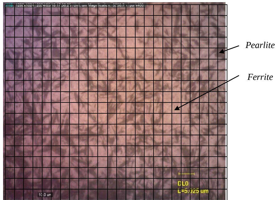
Gambar 6. Hasil Pengujian Variasi Holding Time 60 Menit
