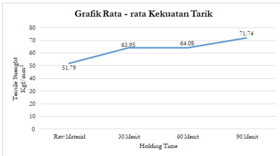
Gambar 2. Grafik Hubungan Tensile Strenght Uji Tarik dengan Variasi Holding Time
