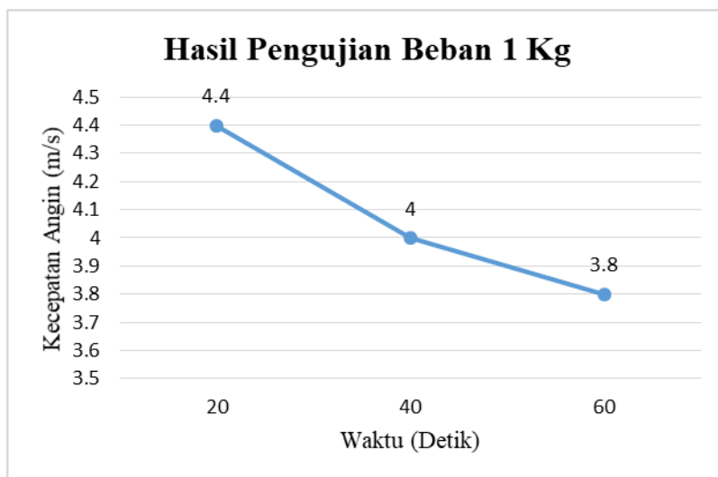
Gambar 2. Grafik Hasil Pengujian Sampah Beban 1 Kg (Sumber : Muhammad Naufal Ramadhani., 2024)
