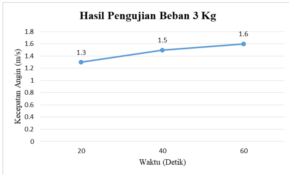
Gambar 4. Grafik Hasil Pengujian Sampah Beban 3 Kg (Sumber : Muhammad Naufal Ramadhani., 2024)
