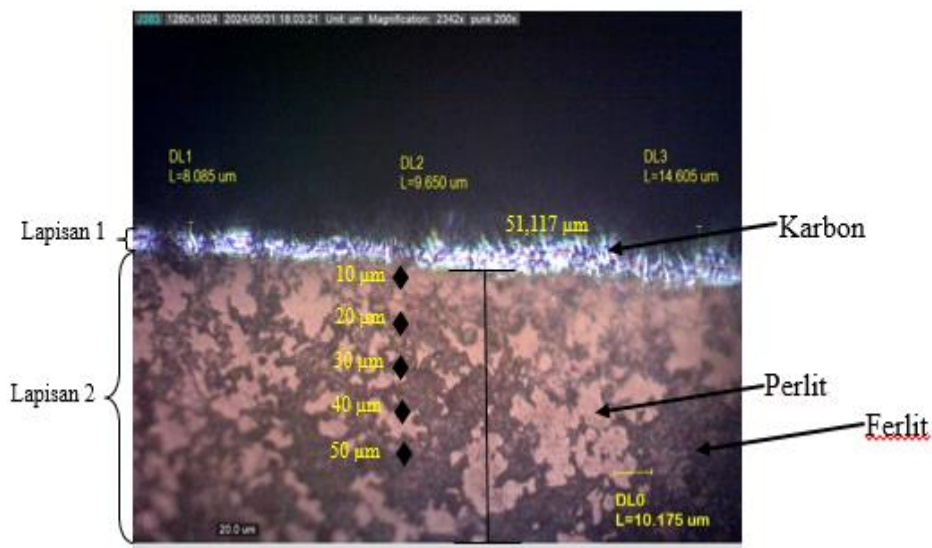
Gambar 2. Ketebalan lapisan baja AISI 1050 hasil proses karburisasi dengan menggunakan laju aliran gas 20 cm 3 /min
