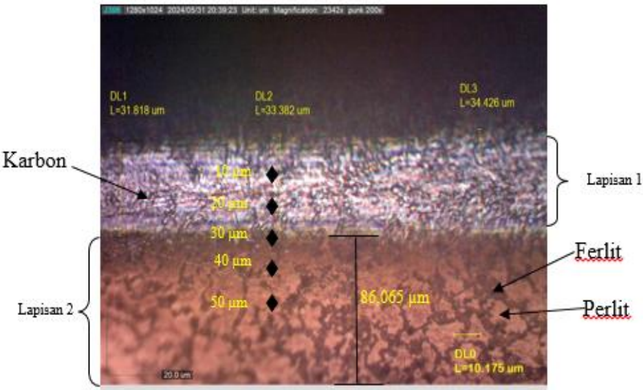
Gambar 3. Ketebalan lapisan baja AISI 1050 hasil proses karburisasi dengan menggunakan laju aliran gas 40 cm 3 /min Gambar 3 menunjukkan material Baja AISI 1050 temperatur 700°C dengan variasi Laju Aliran Gas penahanan 1 jam dilakukan perlakuan panas karburisasi dengan perbesaran 200X terjadi penambahan lapisan karbon pada garis ke 1 Tebal lapisan 31.818 . garis ke 2 Tebal lapisan 33.382, garis ke 3 Tebal lapisan 34.426, dalam satuan mikron (μm).
