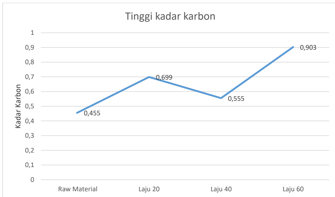
Gambar 7. Grafik perbandingan kadar karbon
