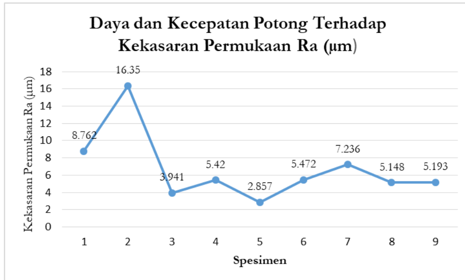
Gambar 3. Grafik daya dan kecepatan pemotongan terhadap kekasaran permukaan Ra (µm)
