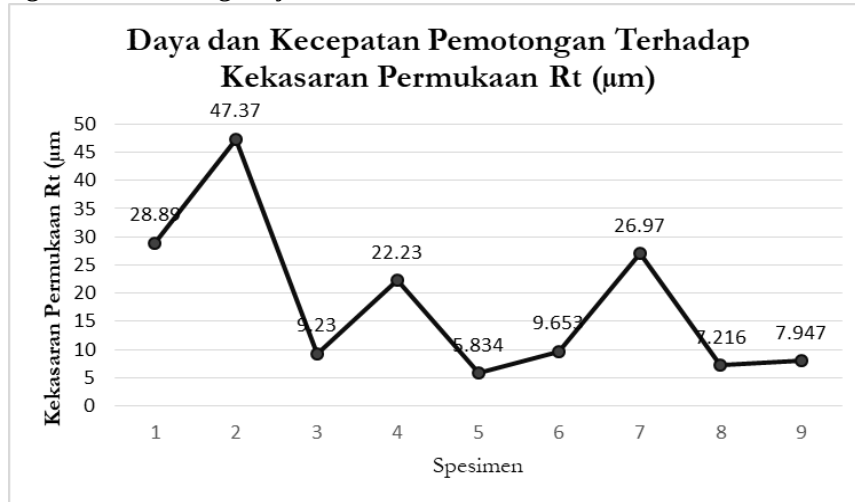
Gambar 4. Grafik daya dan kecepatan pemotongan terhadap kekasaran permukaan R_t ( \mu\text{m} )
