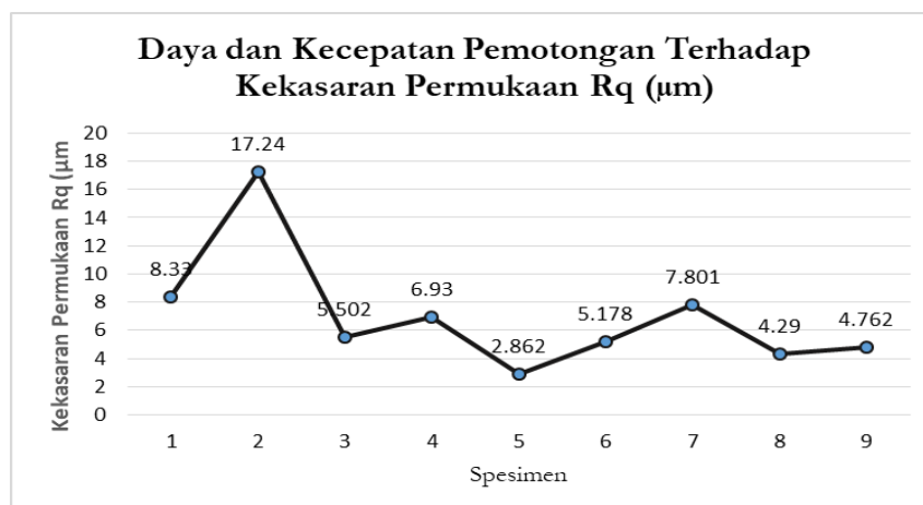
Gambar 5. Grafik daya dan kecepatan pemotongan terhadap kekasaran permukaan R_q ( \mu\text{m} )
