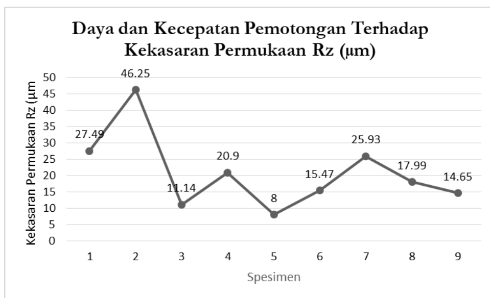
Gambar 6. Grafik daya dan kecepatan pemotongan terhadap kekasaran permukaan Rz ( \mu\text{m} )
