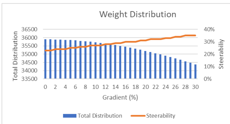
Gambar 4 berat total terhadap performa pada gradient 1% - 30%
