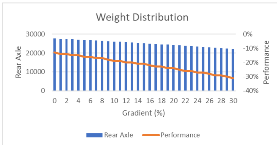
Gambar 3 berat rear axle terhadap performa pada gradient 1% - 30%
