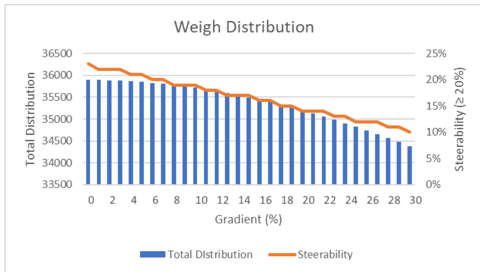
Gambar 7 Grafik berat total terhadap performa pada gradient 1% - 30%
