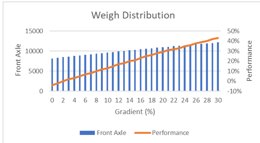
Gambar 2 berat front axle terhadap performa pada gradient 1% - 30%
