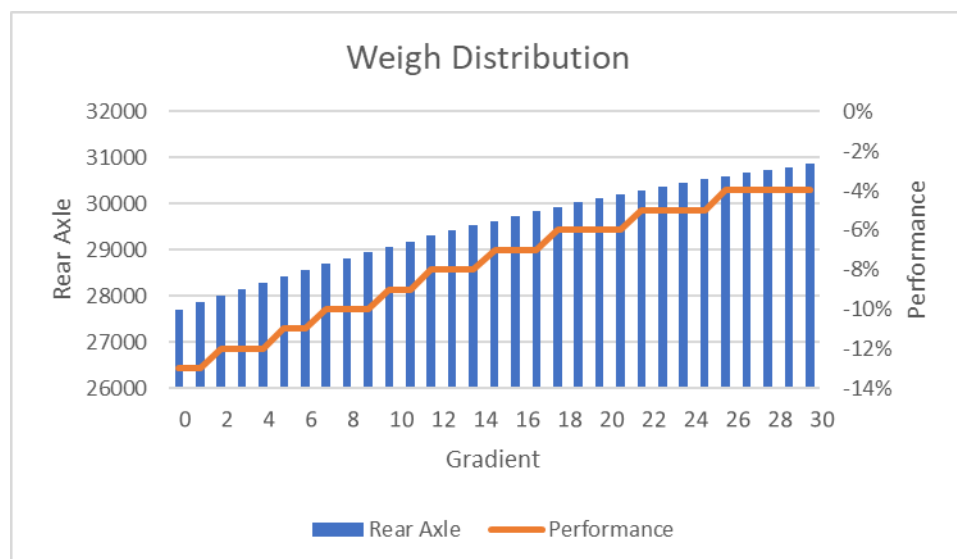
Gambar 6 berat rear axle terhadap performa pada gradient 1% - 30%
