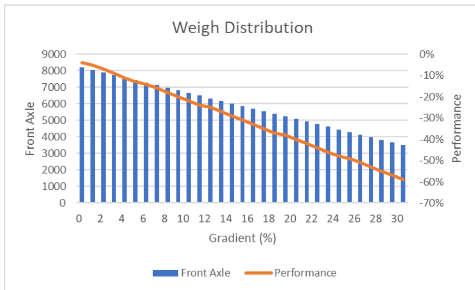
Gambar 5 berat front axle terhadap performa pada gradient 1% - 30%
