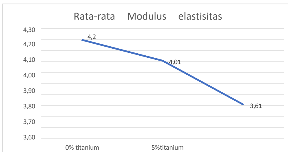
Grafik 2. Modulus Elastisitas
