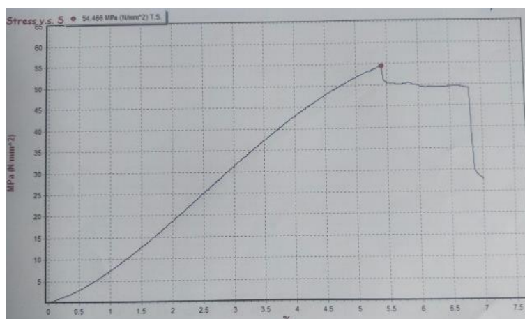
Gambar 15 Grafik Spesimen 4
