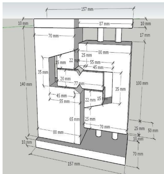
Gambar 1 Konsep Desain
