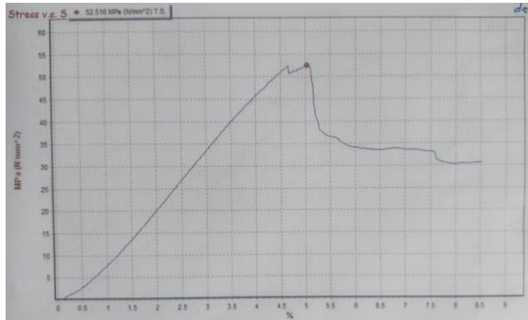
Gambar 16 grafik spesimen 5
