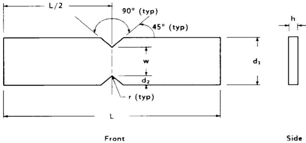
Gambar 8 Ukuran spesimen
