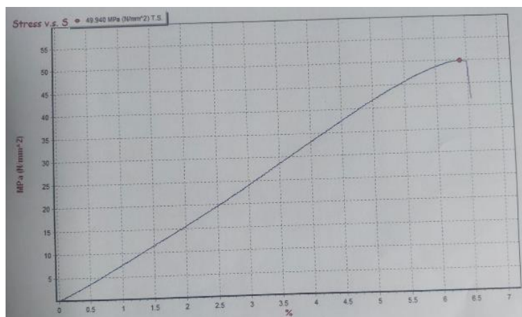
Gambar 12 Grafik Spesimen 1
