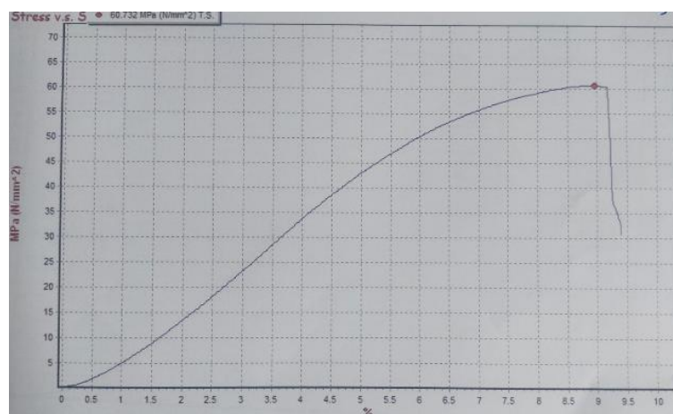
Gambar 14 Grafik Spesimen 3
