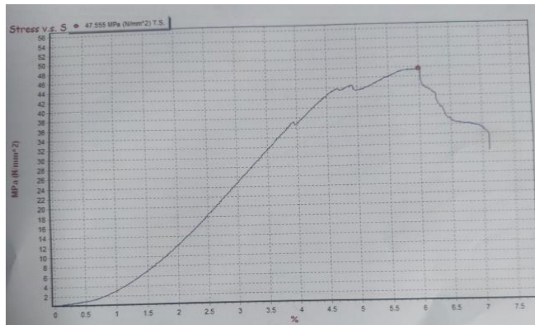
Gambar 13 Grafik Spesimen 2
