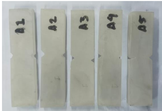
Gambar 10 Spesimen uji
