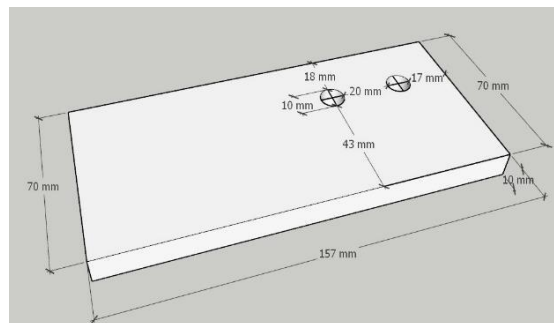
Gambar 6 base plat
