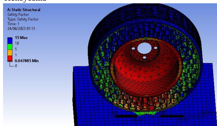
Gambar 13. Nilai faktor keamanan ban tanpa udara tipe spokes honeycomb
