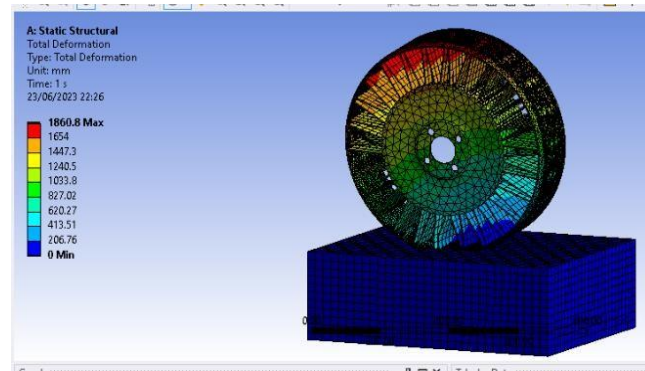
Gambar 8. Nilai deformasi ban tanpa udara tipe spokes twell
