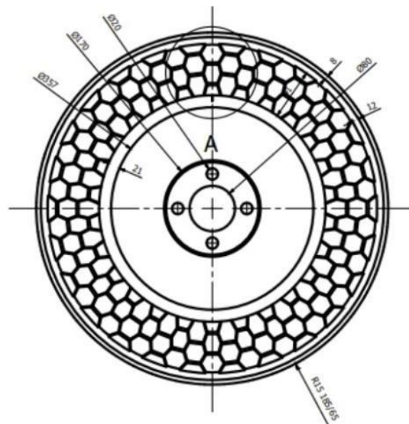
Gambar 5. Dimensi Ban tanpa udara tipe honeycomb
