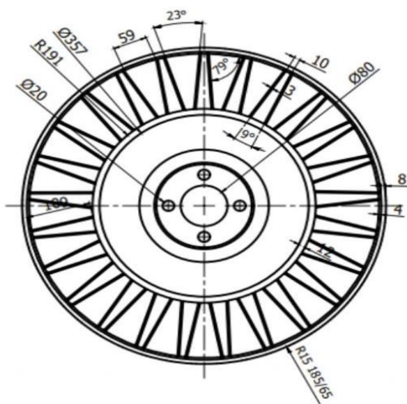
Gambar 2. Ban tanpa udara tipe tweel
