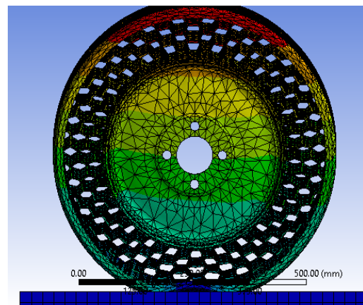
Gambar 15. Hasil simulasi deformasi ban tanpa udara tipe spokes honeycomb
