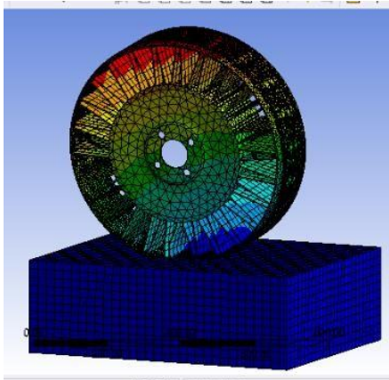
Gambar 14. Hasil simulasi deformasi ban tanpa udara tipe spokes tweel.
