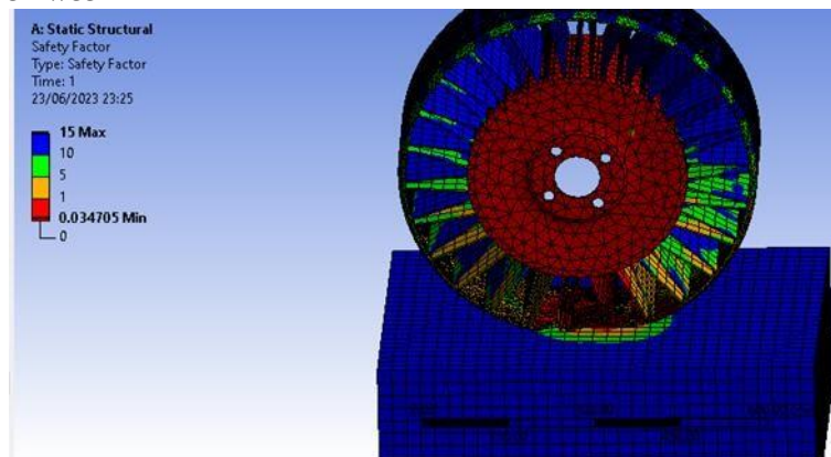
Gambar 12. Nilai faktor keamanan ban tanpa udara tipe spokes tweel
