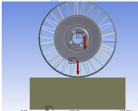
Gambar 7. Letak titik pembebanan dan titik support
