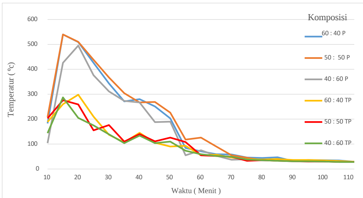
Gambar 5. Hubungan Variasi Komposisi Briket Pada Laju Pembakaran
