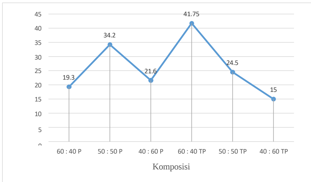
Gambar 7. Grafik Kadar Abu Terhadap Sampel
