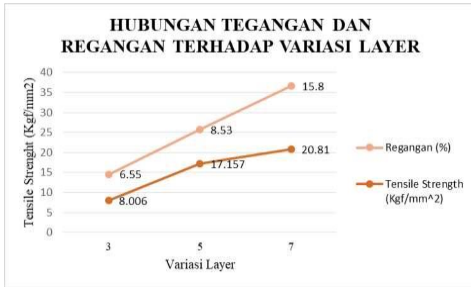
Gambar 2. Grafik Regangan Terhadap Variasi Layer Komposit
