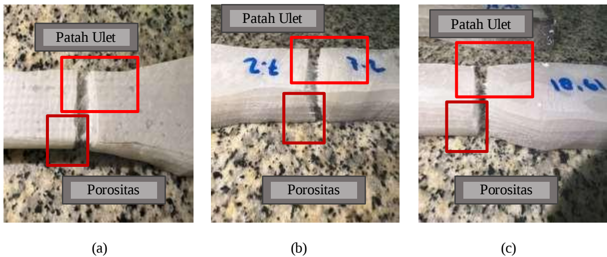
Gambar 7. Spesimen Hasil Uji Strukt Makro
