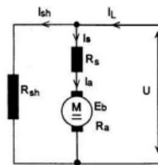
Gambar 8. Rangkaian Motor Kompon Panjang
