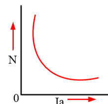
Gambar 5. Kurva Karakteristik n/I_a
