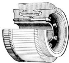
Gambar 13. Komutator Motor DC
