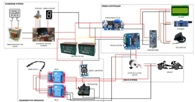
Gambar 16. Wiring Diagram
