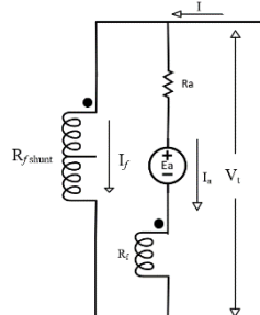
Gambar 7. Rangkaian Ekuivalen Motor Kompon
