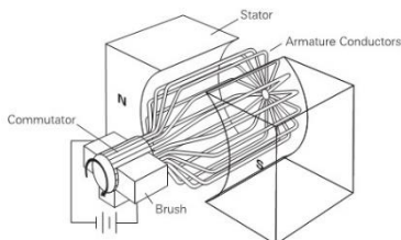
Gambar 14. Sikat Motor DC
