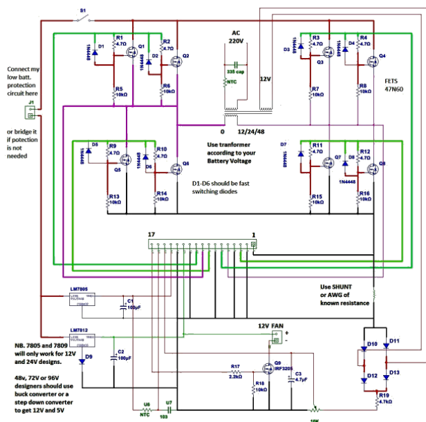
Gambar 15. Perancangan Desain Inverter PWM Sine Wave
