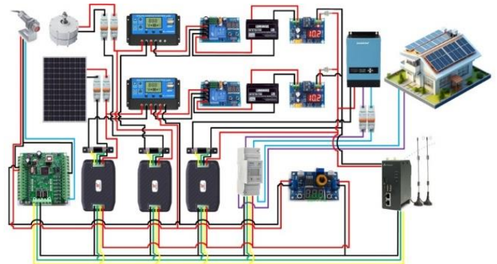
Gambar 14. Perancangan Pembangkit Listrik Pikohidro dan PLTS
