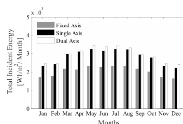
Gambar 4. Perhitungan Energi Bulanan Untuk Berbagai Sistem Pelacakan
