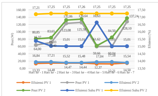
Gambar 19. Grafik Efisiensi & Daya Panel Surya
