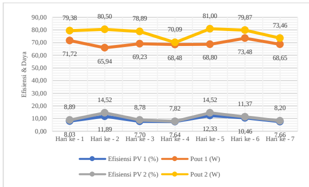
Gambar 18. Grafik Efisiensi & Daya Panel Surya
