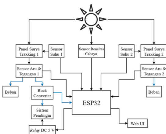
Gambar 16. Blok Diagram Alat
