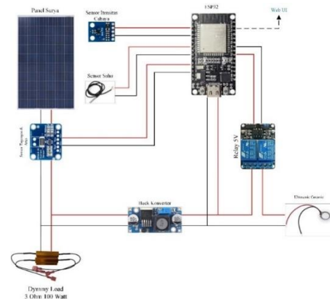
Gambar 17. Perancangan Perangkat Keras
