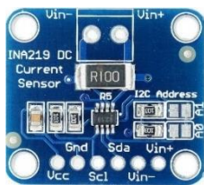
Gambar 8. Sensor Tegangan dan Arus
