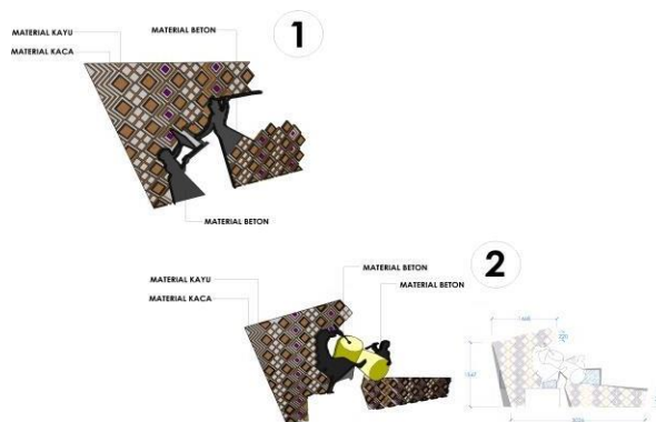
Gambar 14. Detail arsitektural
