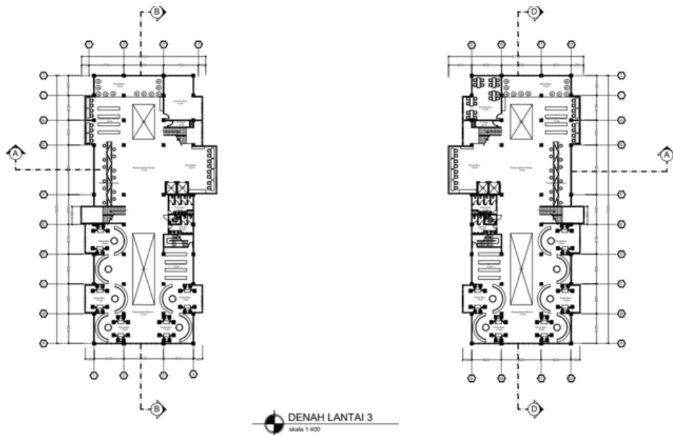
Gambar 17. lantai 3
