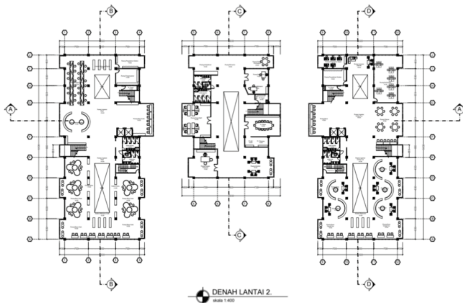
Gambar 16. lantai 2 Sumber: Dokumen Pribadi, 2023
