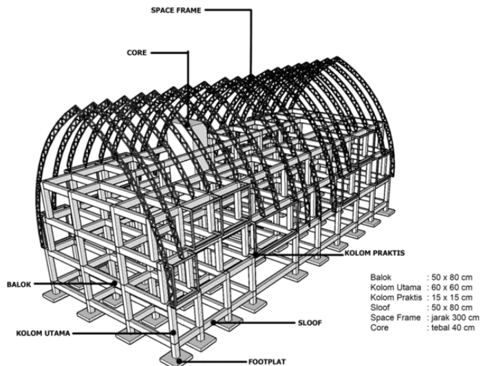
Gambar 6. Konsep Struktur
