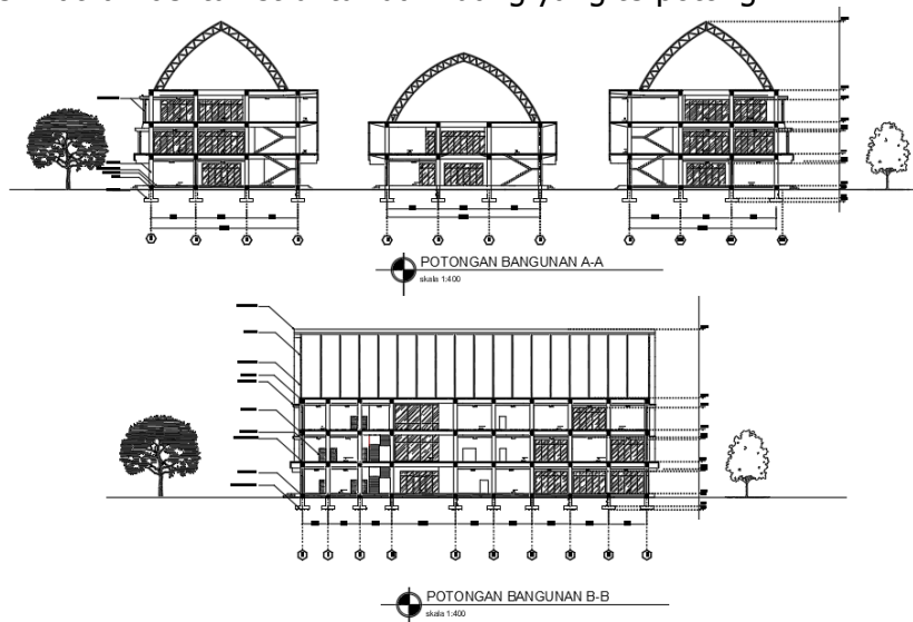
Gambar 19. Potongan Bangunan
