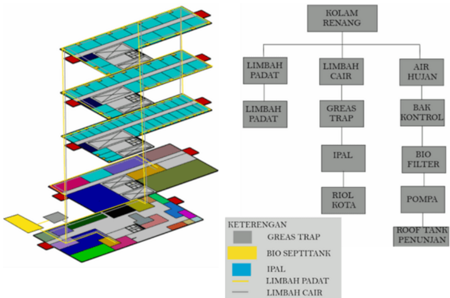
Gambar 8. Konsep Air Kotor
