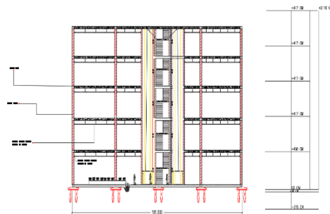
Gambar 13. Potongan A-A
