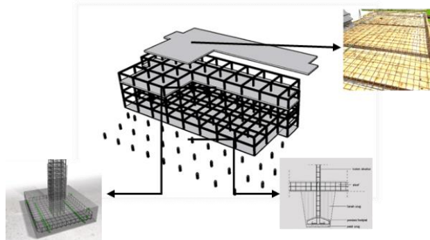
Gambar 6. Konsep Struktur
