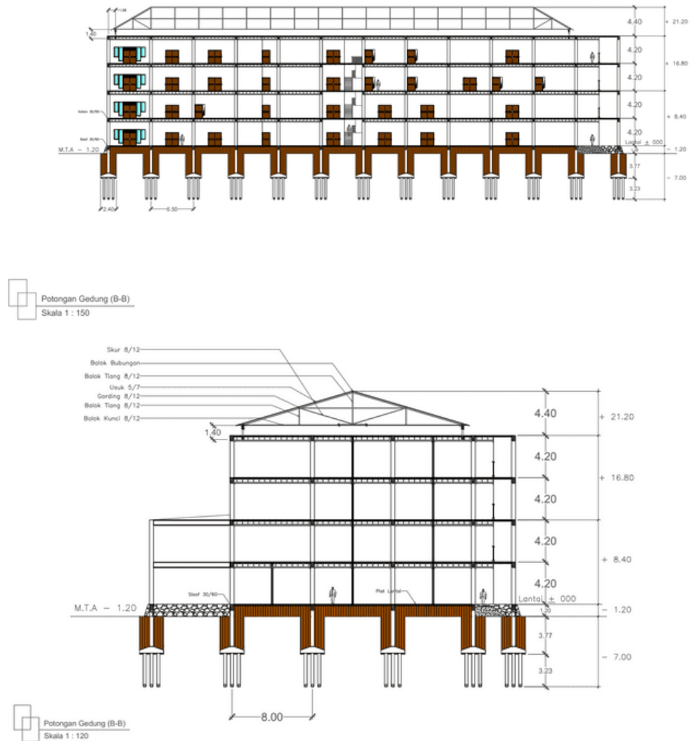
Gambar 20. Gambar Potongan
