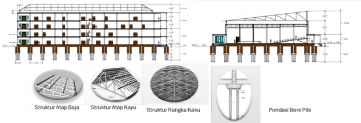
Gambar 14. Struktur Pada Bangunan Sumber: Data Pribadi, 2023
