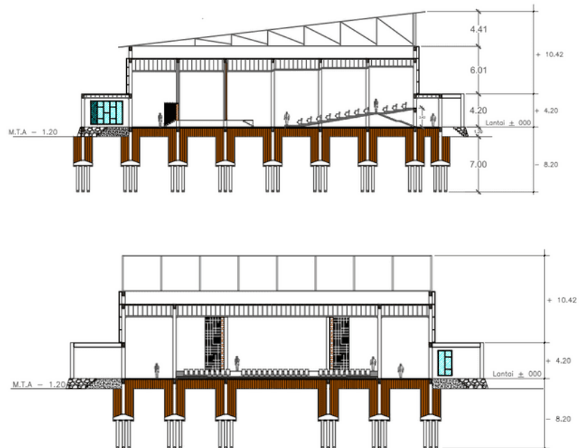
Gambar 21. Gambar Potongan Sumber: Data Pribadi, 2023
