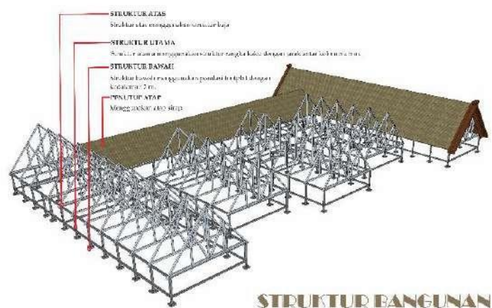
Gambar 12. Konsep Struktur
