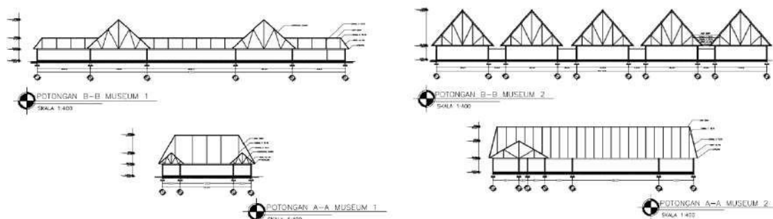
Gambar 18. Potongan bangunan Sumber : Analisis, 2023
