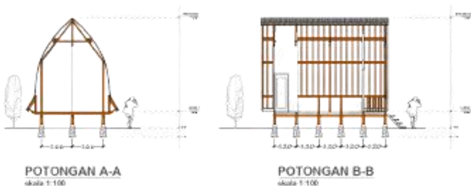
Gambar 19. Potongan Cottage
