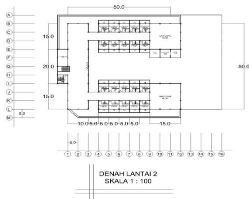
Gambar 13. Konsep Tataan Ruang Lantai 2 Sumber: Gambar Pribadi.
