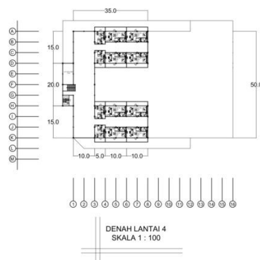
Gambar 15. Konsep Tatahan Ruang Lantai 4
