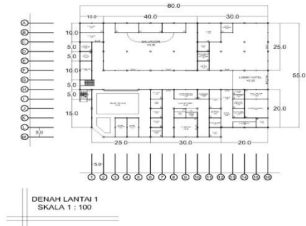
Gambar 12. Konsep Tataan Ruang Lantai 1 Sumber: Gambar Pribadi.
