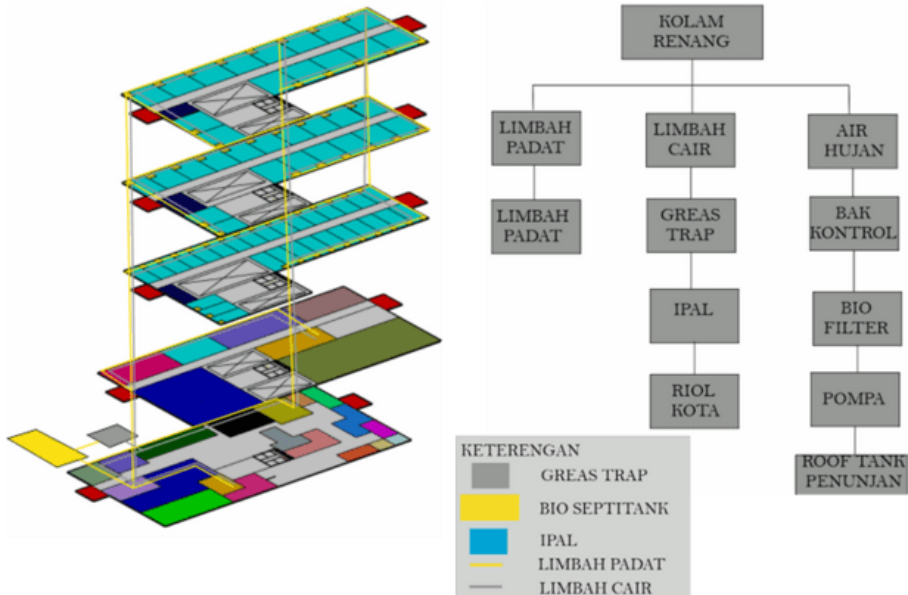
Gambar 8. Konsep Air Kotor
