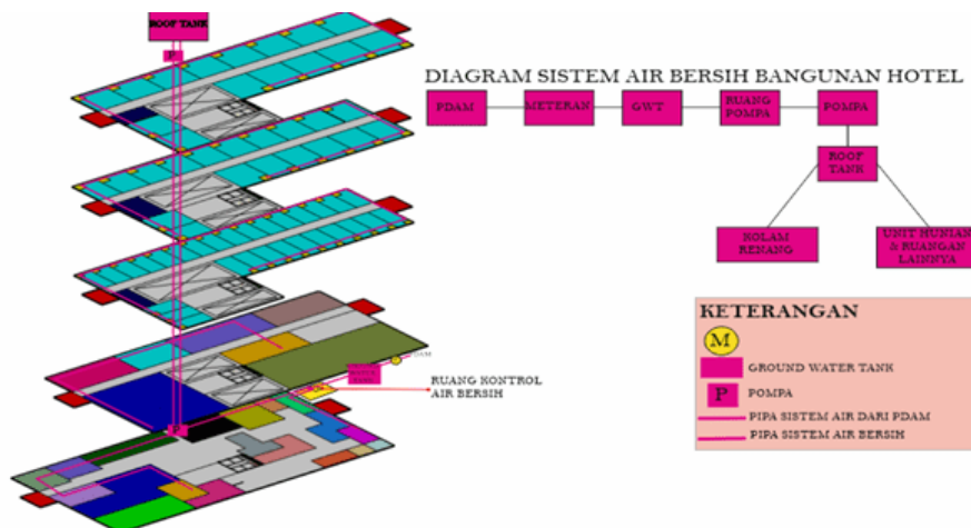
Gambar 7. Konsep Air Bersih
