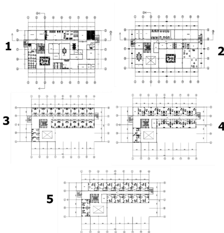
Gambar 12. Denah Lantai 1-5 Sumber : Analisis, 2023
