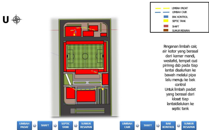
Gambar 9. Rancangan Air Kotor Sumber : Dokumen Pribadi, 2023
