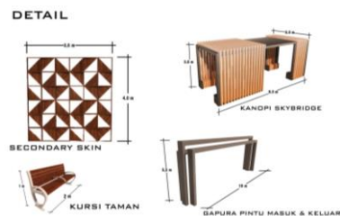
Gambar 17. Detail Sumber : Analisa Pribadi, 2023
