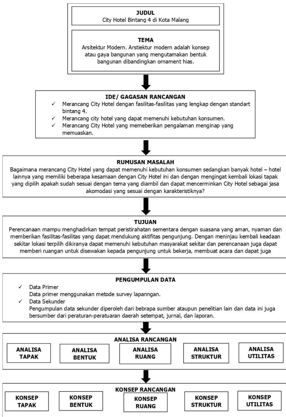
Gambar 3. Metode Perancangan
