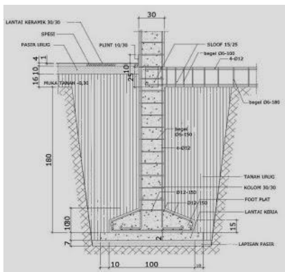
Gambar 9 : Sub Structure Sumber : Data Pribadi
