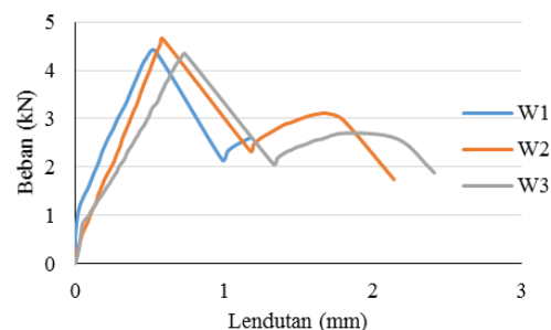
Gambar 10. Grafik hubungan beban dan lendutan benda uji lentur menggunakan perkuatan
