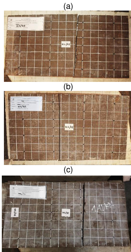
Gambar 11. (a) Pola kerusakan benda uji W1, (b) Pola kerusakan benda uji W2, (c) Pola kerusakan benda uji W3
