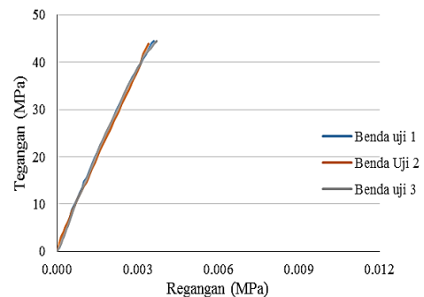
Gambar 5. Grafik hubungan tegangan dan regangan umur 28 hari
