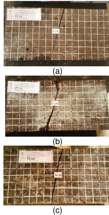
Gambar 9. (a) Pola kerusakan benda uji L1, (b) Pola kerusakan benda uji L2, (c) Pola kerusakan benda uji L3
