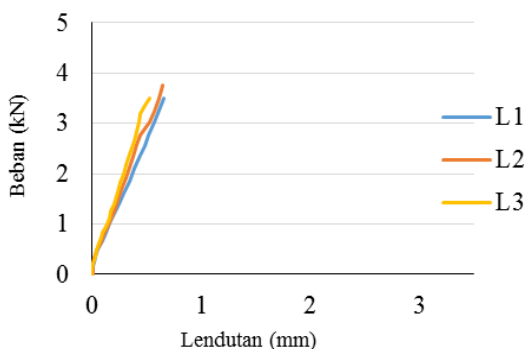
Gambar 8. Grafik hubungan beban dan lendutan benda uji lentur tanpa perkuatan
