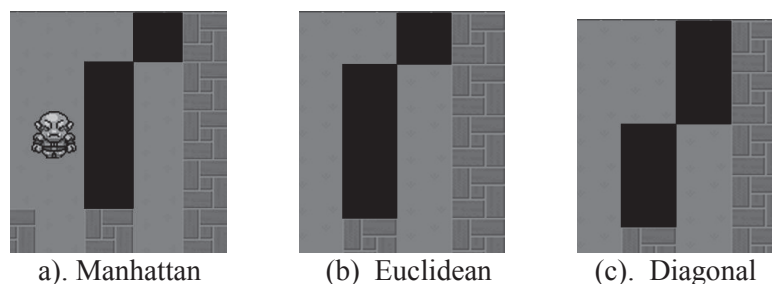
Gambar 4. Pengujian Heuristik
