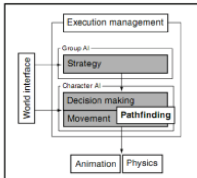
Gambar 3. Letak pathfinding dalam game AI model [1]
