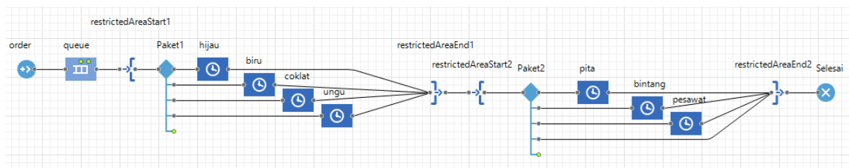
Gambar 2. Penerapan Simulasi pada Anylogic
